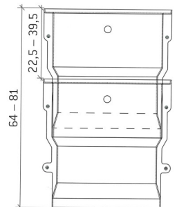
Plaatsing bij opstand met afgesneden bevestigingsogen (in cm)
