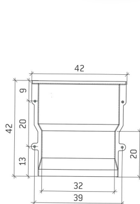
Afmetingen verluchtingsschacht (in cm)
