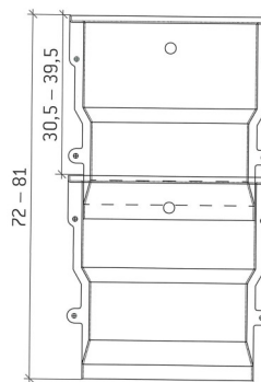
Plaatsing bij opstand met bevestigingsogen (in cm)
